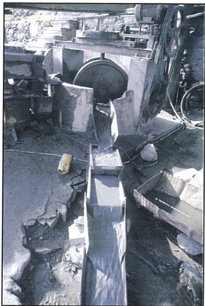
17. Molino Trapiche con plancas amalgamadoras (Coop. La Suerte, Bolivia)
