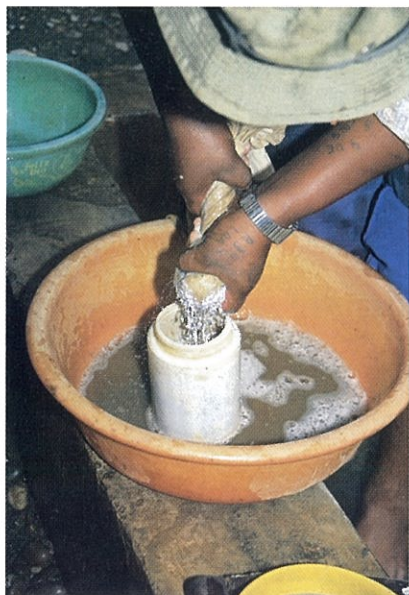
23. Exprimir el mercurio líquido de la amalgama manualmente por un trapo (Coop. Tupara, Bolivia)
