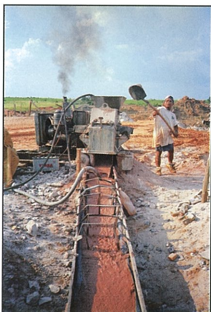
18. Molino a martillos con planchas amalgamadoras (San Simón, Bolivia)
