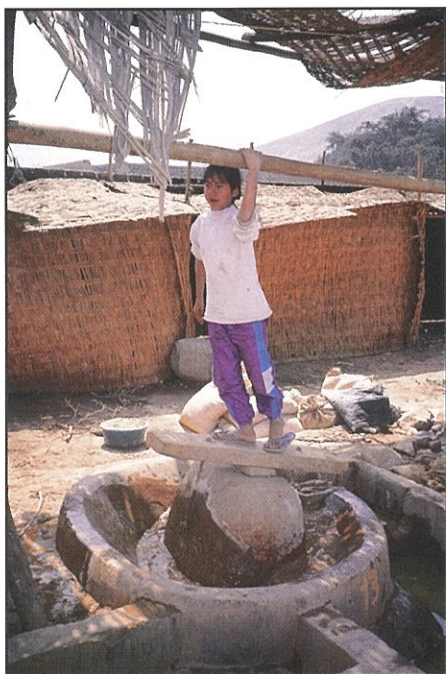
20. Molino/amalgamador de piedra (típicamente trabajo de niños o mujeres) (Nazca, Perú)
