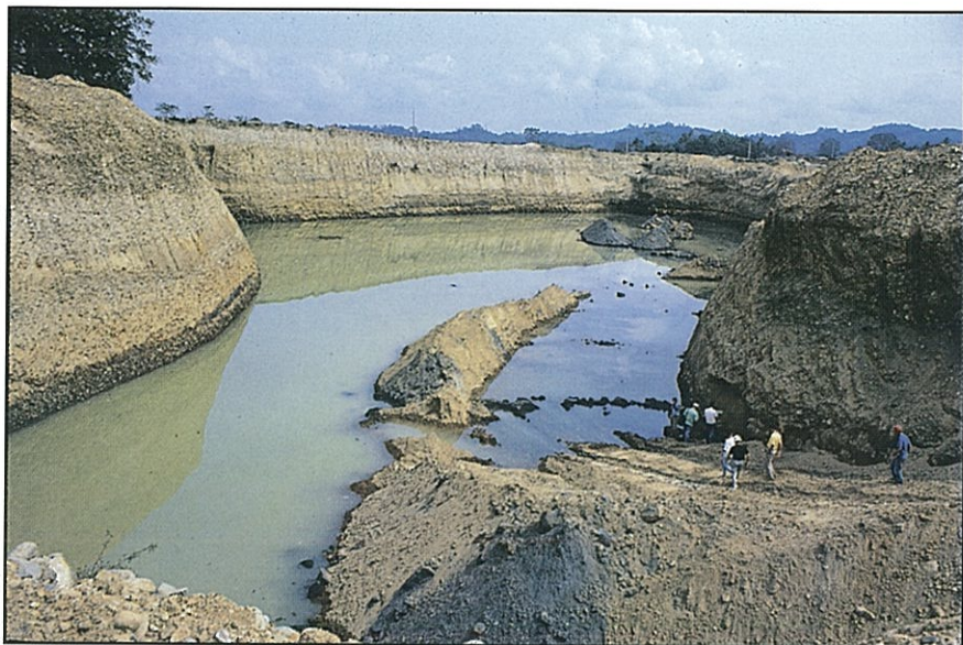
5. Minería aluvial: lagunas restantes (Coop. Tupara, Bolivia)
