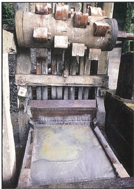
19. Molino a piones con planchas amalgamadoras (Mina Los Guavos, Nariño, Colombia)
