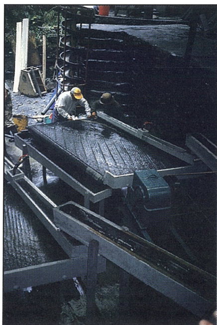
31. Canaletas con diferentes pisos (alfombras, metal expandido) para diferentes tamaños de carga clasificados por un tromel en la salidad de un molino a bolas (Coop. La Libertad, Bolivia)
