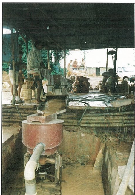
22. Amalgamación en concentradores centrífugos (Km 88, Venezuela)
